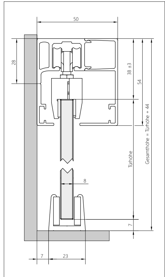
Vertikalschnitt
