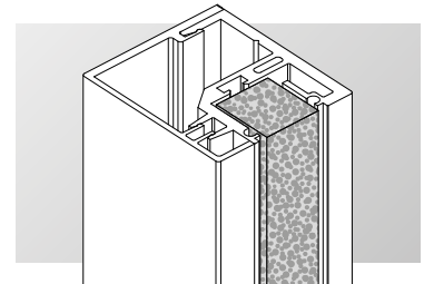
Anschlagkasten für Holztüren – mit Dichtungsband aus Schaumstoff.
