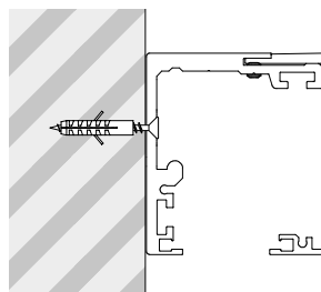
Laufschienen – entweder zur Decken- oder Wandmontage vorgebohrt und gesenkt.
