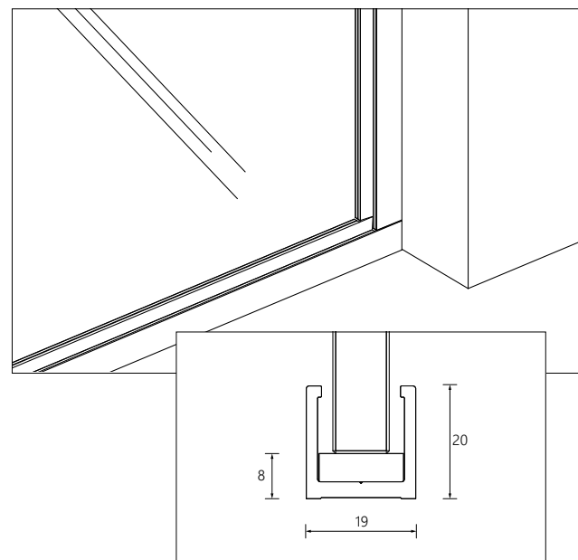
Boden- und Wandanschluss
