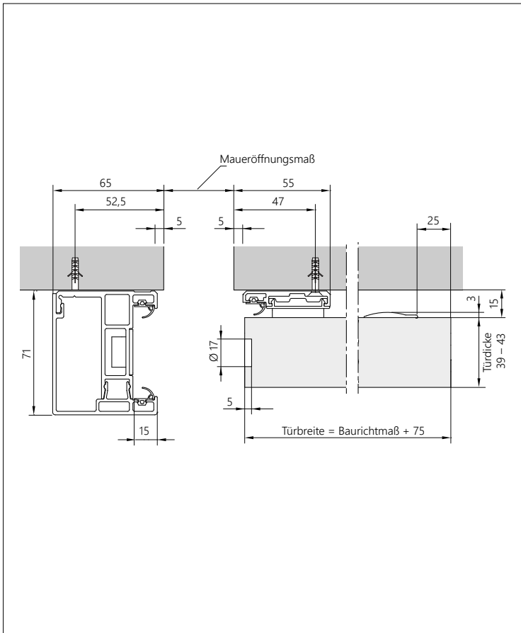
Horizontalschnitt
