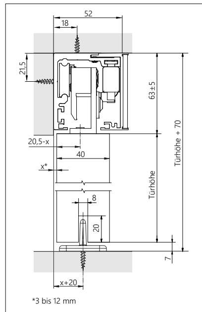
Vertikalschnitt mit Dekorblende
