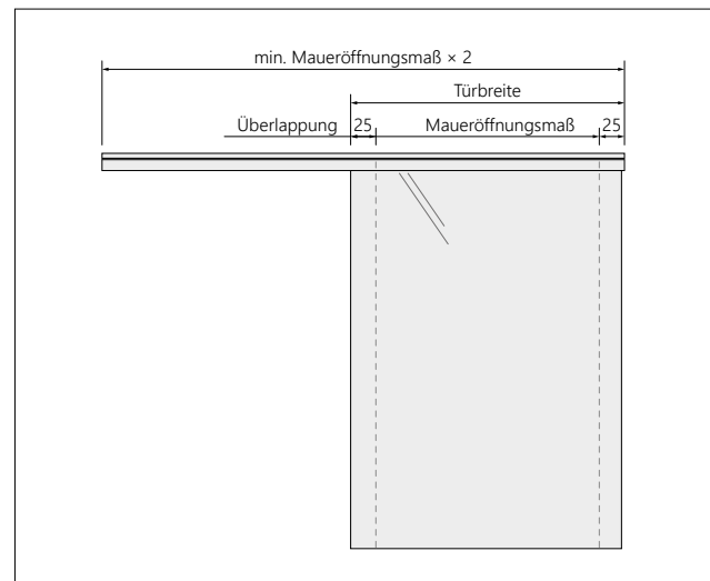
Frontalansichten (Schema)
