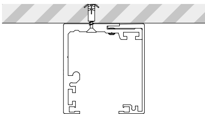
Laufschienen – entweder zur Decken- oder Wandmontage vorgebohrt und gesenkt.
