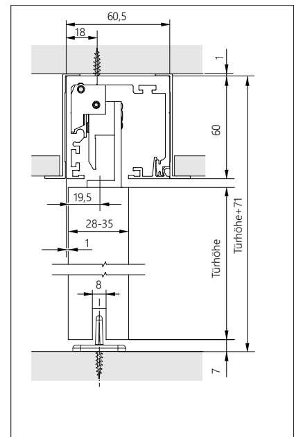
Vertikalschnitt mit integrierter Deckenschiene
