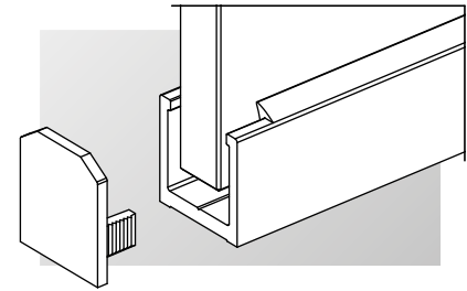
Endkappe für Bodenanschlussprofil
