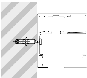
Laufschiene – zur Wandmontage vorgebohrt.
