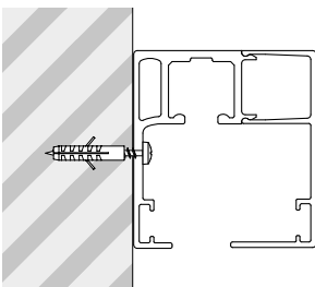
Laufschiene – zur Wandmontage vorgebohrt.
