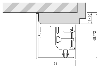
Anschlagkasten auf Zarge
