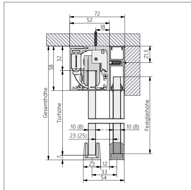
Vertikalschnitt
