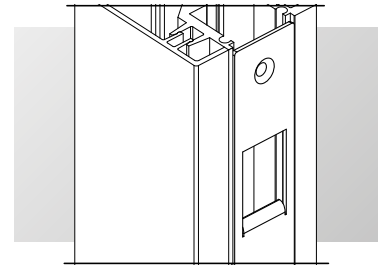
Schließblech – stufenlos verstellbar
