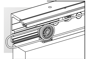
Seilzug-System für Holztüren
