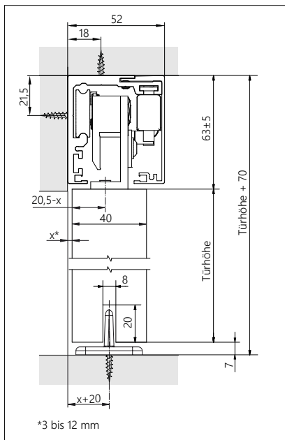
Vertikalschnitt Wand-/Deckenmontage
